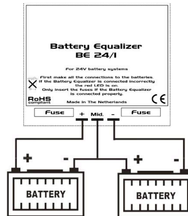
24 Volt battery system
